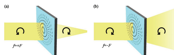
图4 不同偏振光下液晶偏振透镜的作用效果图
