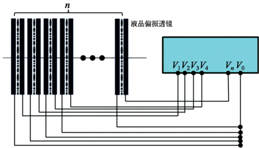
图 6 液晶偏振透镜串联变焦结构示意图
