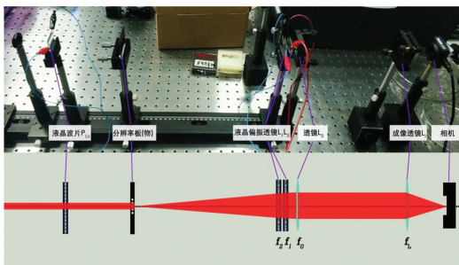
图 12 液晶偏振变焦透镜组成像实验光路图
