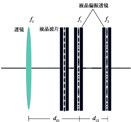
图 7 液晶偏振变焦透镜组结构示意图
