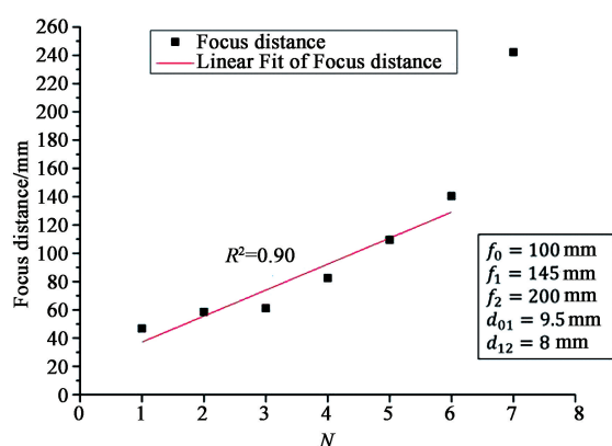
图8 LCPL变焦系统点距离分布图
