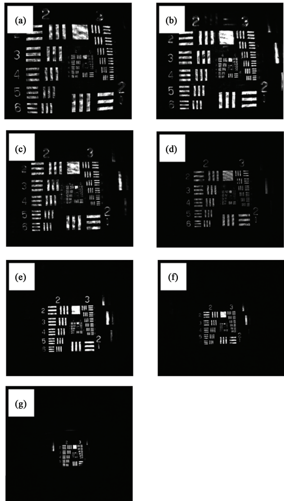
图 13 分辨率板在液晶偏振变焦透镜组不同焦距时的清晰成像图
