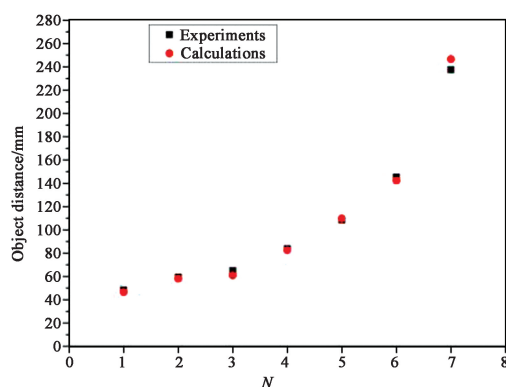
图14 成像距离分布图
