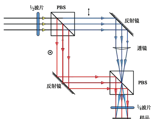
图3 液晶偏振透镜干涉曝光光路
