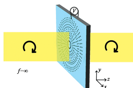
图5 电场作用下液晶偏振透镜光学效果
