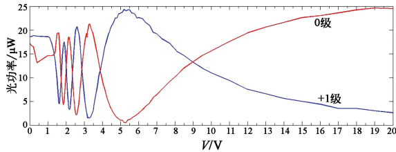
图 11 532 nm 圆偏振光下,液晶偏振透镜的电光特性曲线。
