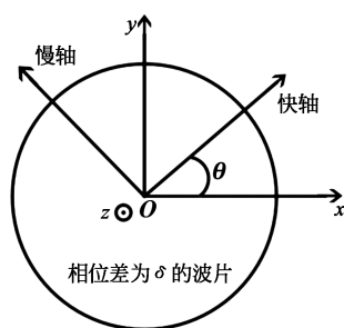
图2 波片琼斯矩阵的推导
