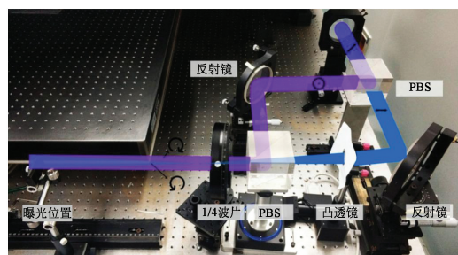
图9 液晶偏振透镜制备光路图
